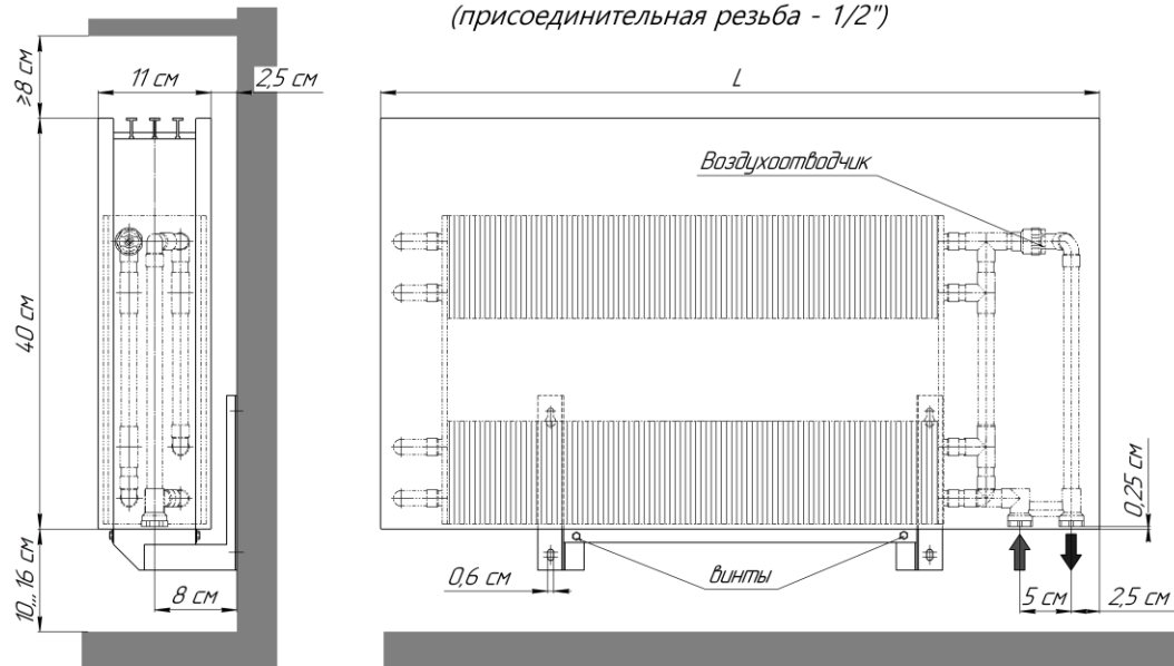
Настенный конвектор "Элегант 110х400-4то Терм Стен прав" с правосторонним нижним подключением (левостороннее - зеркально) с встроенным термоклапаном. (присоединительная резьба - 1/2")
