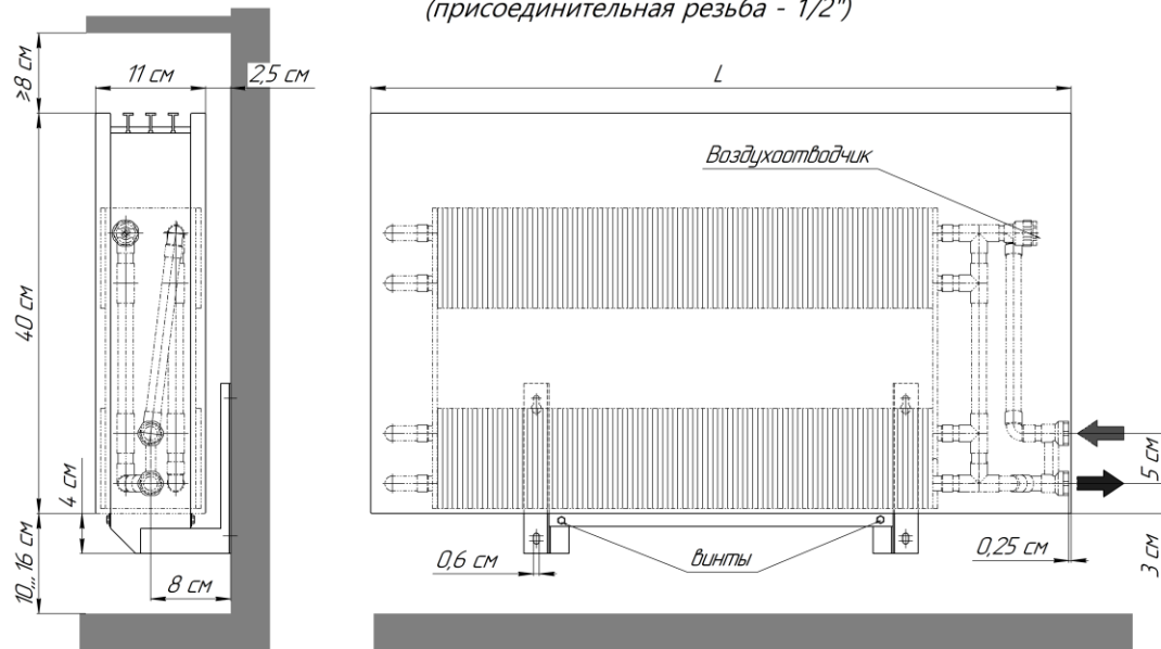
Настенный конвектор "Элегант 110х400 4то бок Стен прав" с правосторонним боковым подключением (левостороннее - зеркально). (присоединительная резьба - 1/2")
